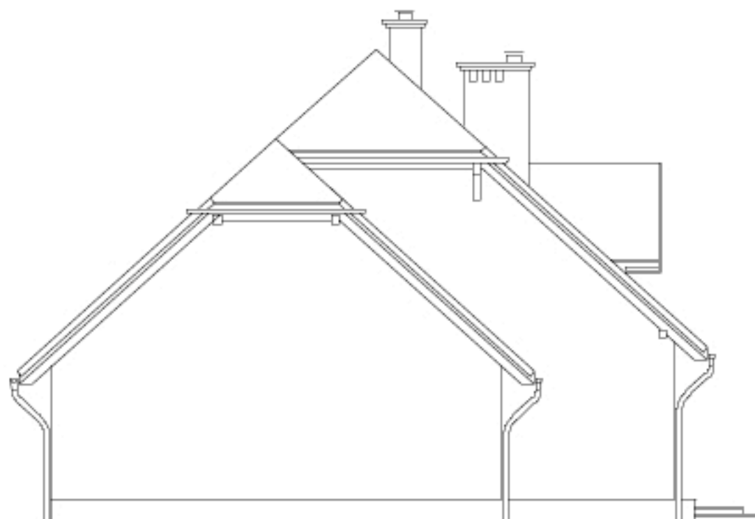
ELEWACJA BOCZNA
